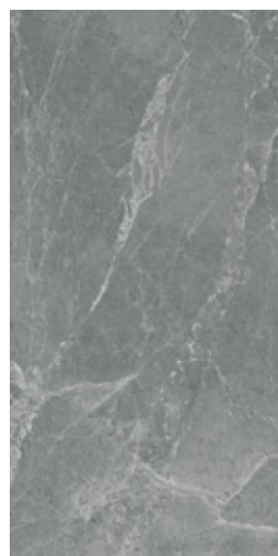
EARTH
