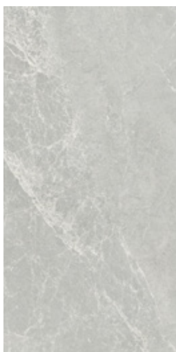
MOON
